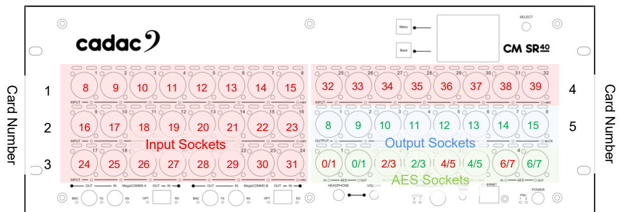
45: Cadac CM-SR40
